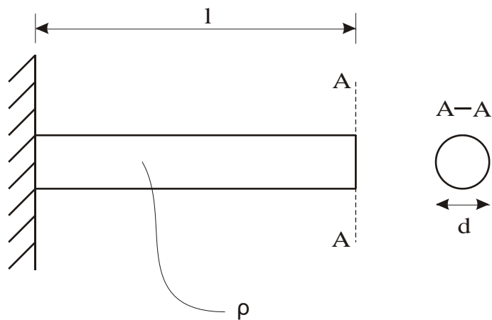
Bild 8: Biegebalken
