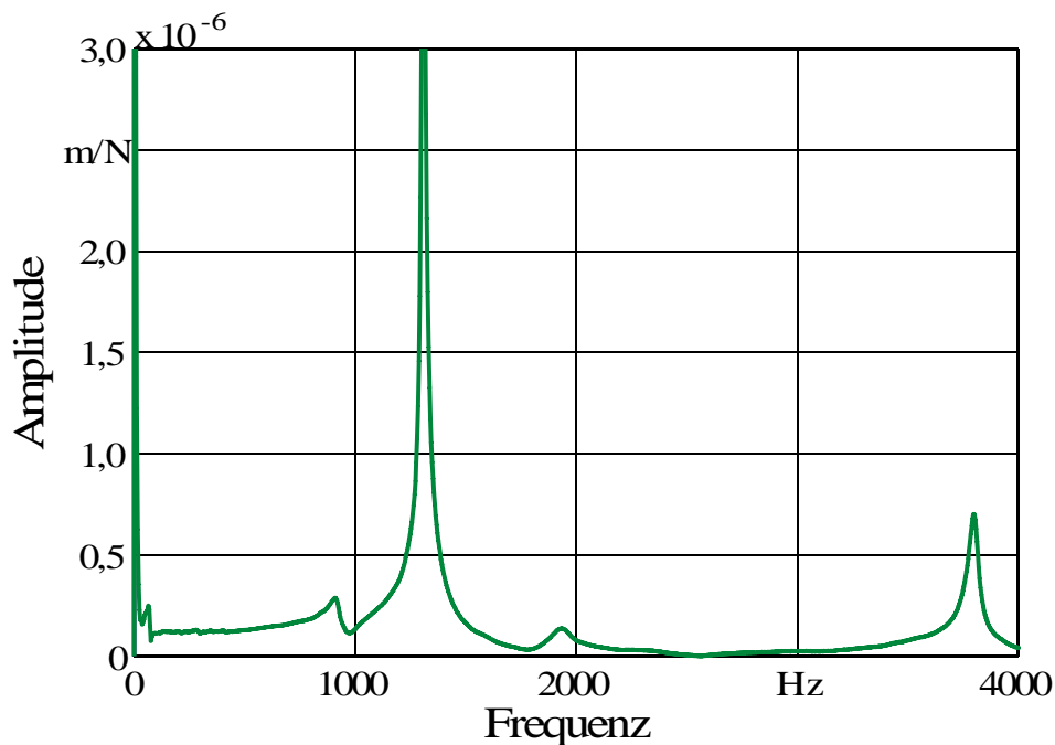
Bild 7: Nachgiebigkeitsfrequenzgang
