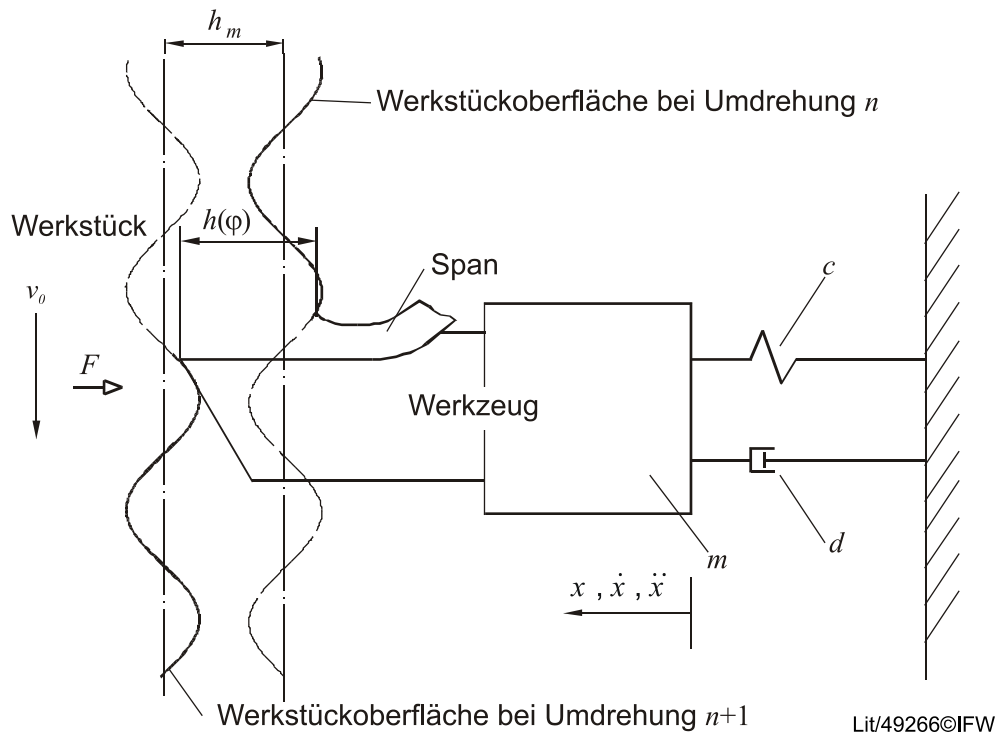
Bild 3: Regeneratives Rattern
